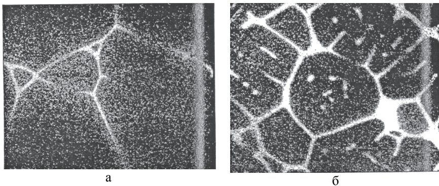
Рис. 7. Ликвация фосфора в а – доперитектическом сплаве с 0,1%С, 0,4% Р; б – перитектическом сплаве с 0,4%С, 1,3%Р; распределение фосфора в K_\alpha излучении. \times 320 по [7].
