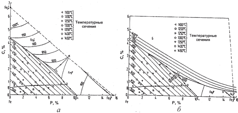
Рис. 5. Изотермы поверхностей ликвидусов Fe-угла метастабильной (а) и стабильной (б) диаграмм Fe-C-P по [13]
