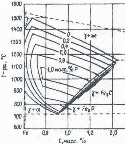
Рис. 5. Изотермы поверхностей ликвидусов Fe-угла метастабильной (а) и стабильной (б) диаграмм Fe-C-P по [13]
