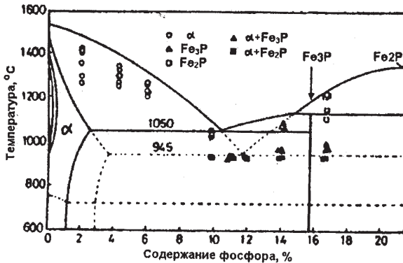
Рис.2. Диаграмма состояния сплавов Fe-P [6]
