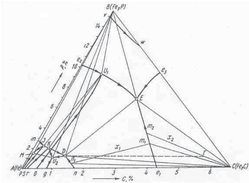
Рис.4. Диаграмма состояния Fe- Fe 3 C- Fe 3 P [9].
