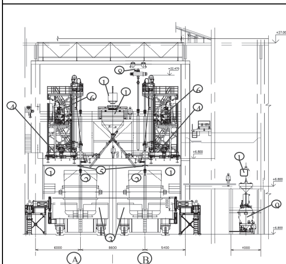
Рис.4. Комплекс десульфурации чугуна (КДЧ) вдуванием гранулированного магния в заливные ковши (290 т) компании CSC (поперечный разрез постов А и В). 1 – камера обработки чугуна; 2 – ковш с жидким чугуном; 3 – подвижный чугуновоз; 4 – устройства ввода фурм в расплав; 5 – фурмы для вдувания магния; 6 – модуль-дозатор зернистого магния; 8 – кран-балка для перемещения и смены фурм; 9 – загрузочный модуль магния; 10 – транспортный контейнер с магнием; 11 – силос сыпучих добавок в ковш (с дозатором); 16 – контейнер с корректирующими добавками.
