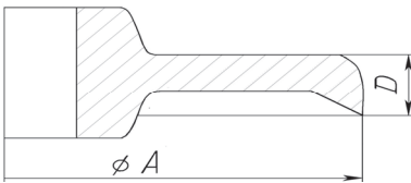
Рис.1 Заготовка для производства колёс и колёсных центров. (Powell-Brett)
