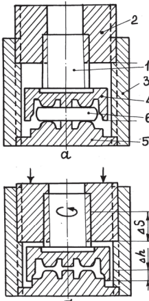
Рис.4. Схема моделирования получения крановых колёс путём осадки с кручением а – начальный момент штамповки; б – окончание штамповки.
