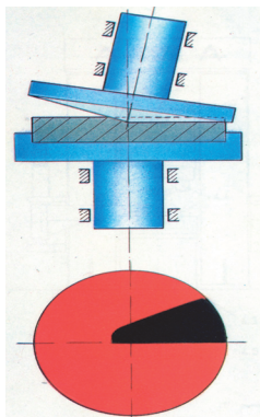
Рис.6. Схема деформирования и конфигурация очага деформации при раскатке на машинах AGW
