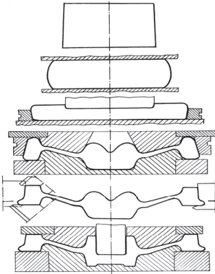
Рис.9. Схема поэтапной деформации колёс в применении к существующим цехам
