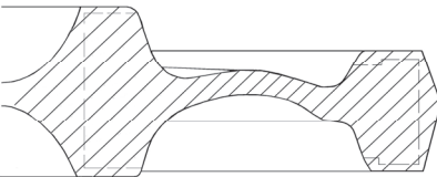
Рис.2. Готовая поковка локомотивного центра. (Powell-Brett)
