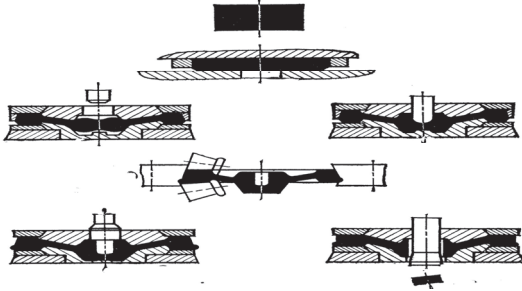
Рис.9. Схема поэтапной деформации колёс в применении к существующим цехам
