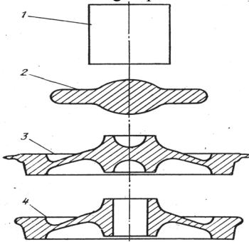
Рис.3.Схема производства колес на заводе фирмы «Chambersburg», США: 1 – заготовка; 2 – осадка и раздача на молоте 11,34 тс; 3 – формовка на молоте 15,87 тс; 4 – прошивка отверстия и обрезка заусенцев
