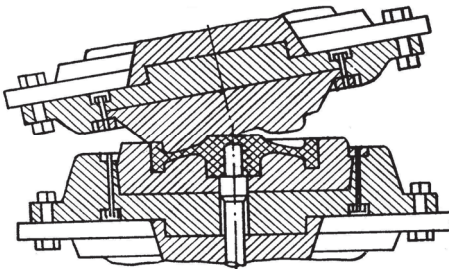
Рис.5.Прокатка колёсных центров в штампах.
