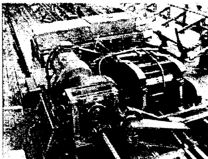
Рис.5. Механизм подачи, установленный на минимально возможном удалении от подвижного очага деформации стана холодной прокатки труб
